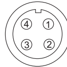
Pinout connettore Binder 712 - 4 pin femmina vista esterna
