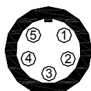
Pinout connettore Binder 712 5 pin femmina vista esterna
