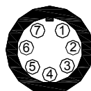
Pinout connettore Binder 712 7 pin femmina vista esterna
