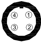
Connettore Binder 712 4 pin femmina vista frontale
